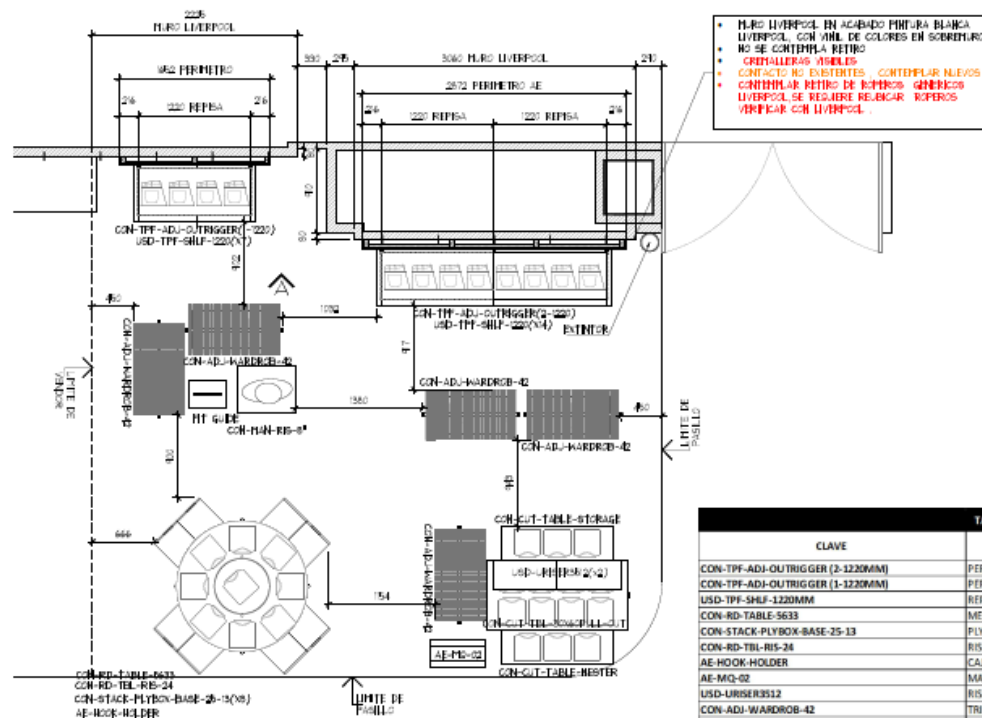
PLANTA MOBILIARIO ESC. 1:50
