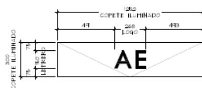
DETALLE LOGO 1 ESC. 1:20
