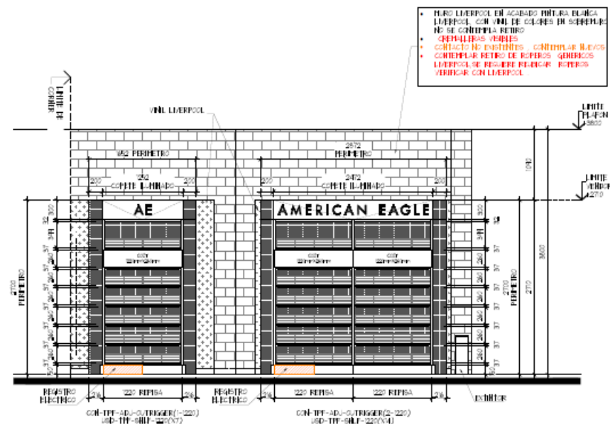
ALZADO A ESC. 1:50
