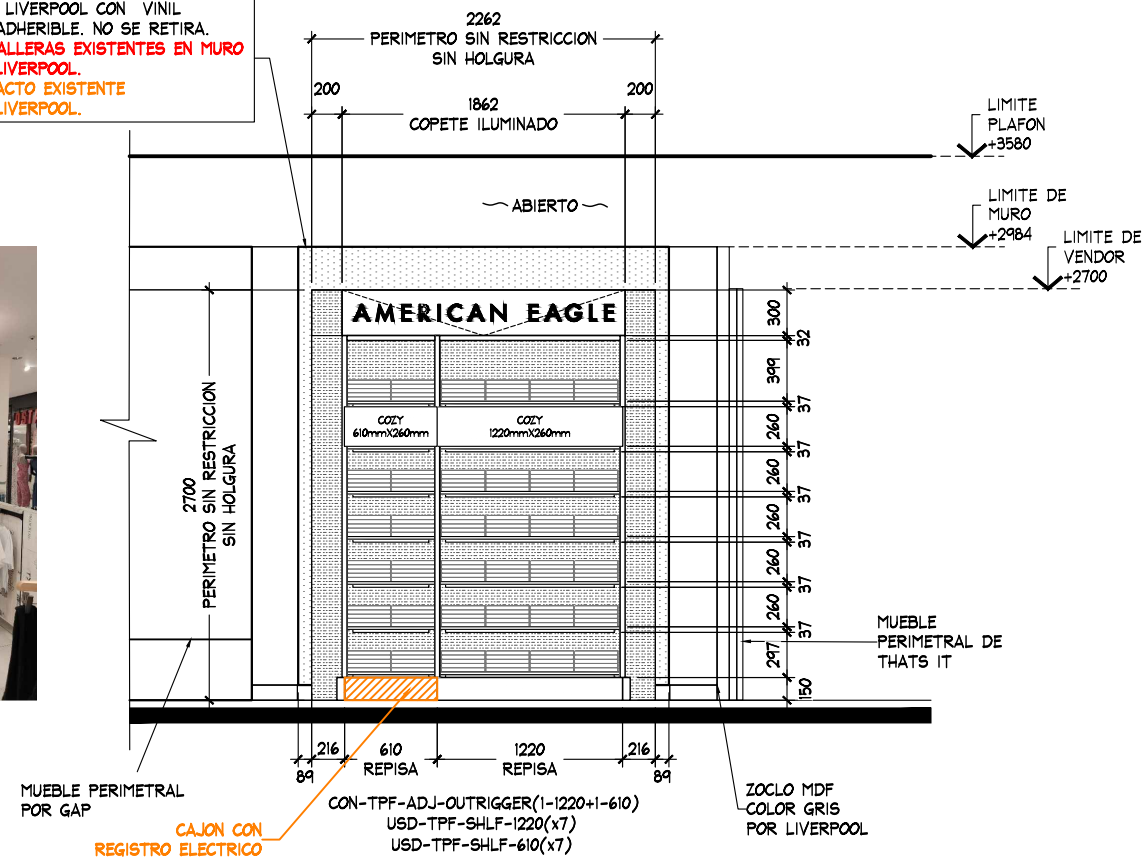
ALZADO A ESC. 1:50
