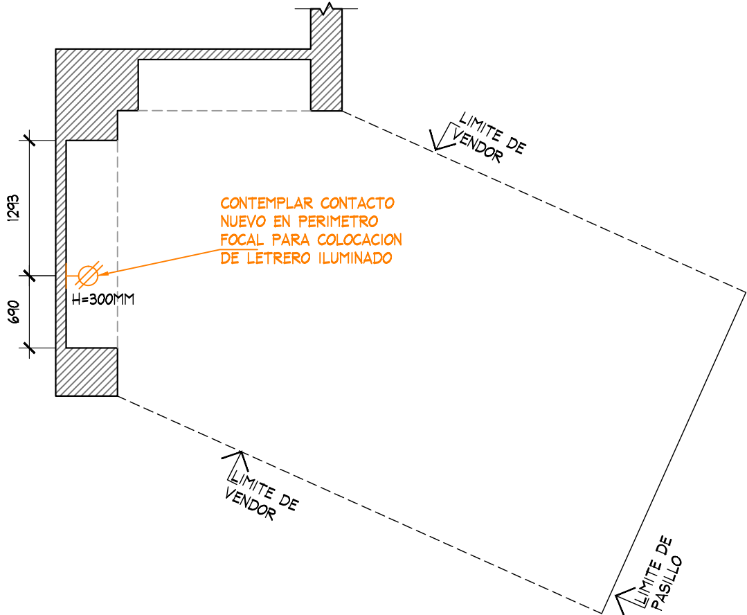
PLANTA DE FUERZA ESC. 1:50
