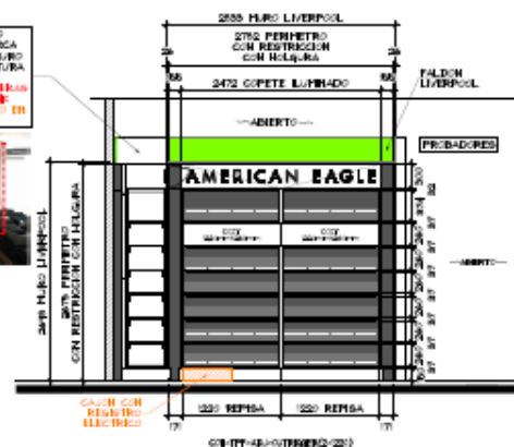
ALZADO C ESC. 1:50
