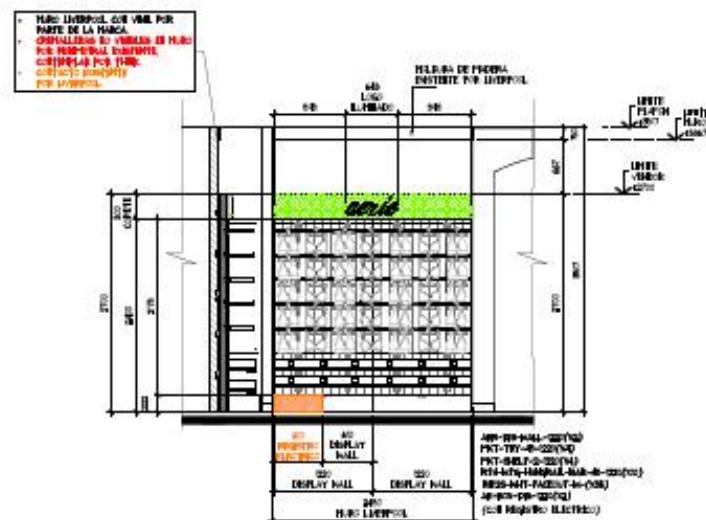
ALZADO A ESC. 1:50
