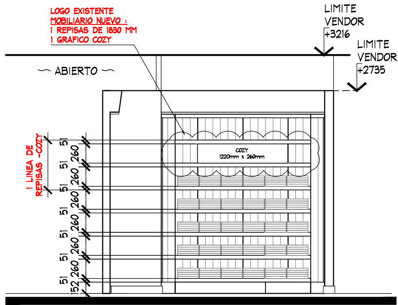
ALZADO B ESC. 1:50
