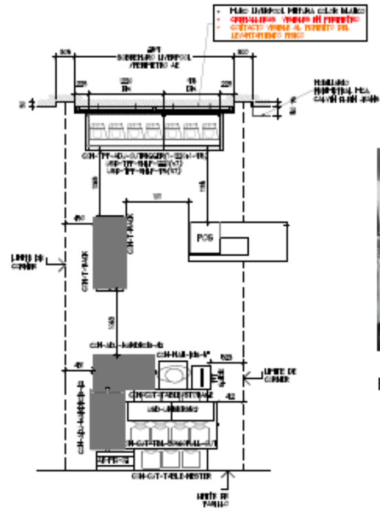
PLANTA ARQUITECTÓNICA ESC. 1:50
