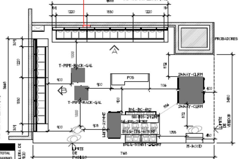
PLANTA ARQUITECTONICA ESC. 1:50
