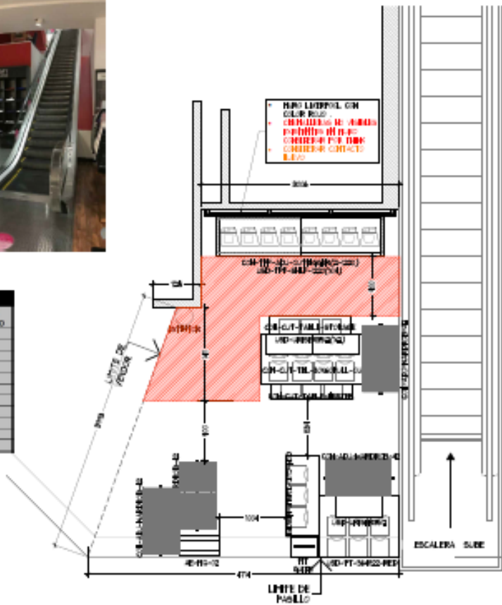
PLANTA DE ALBANILERIA LEVANTAMIENTO ESC. 1:60
