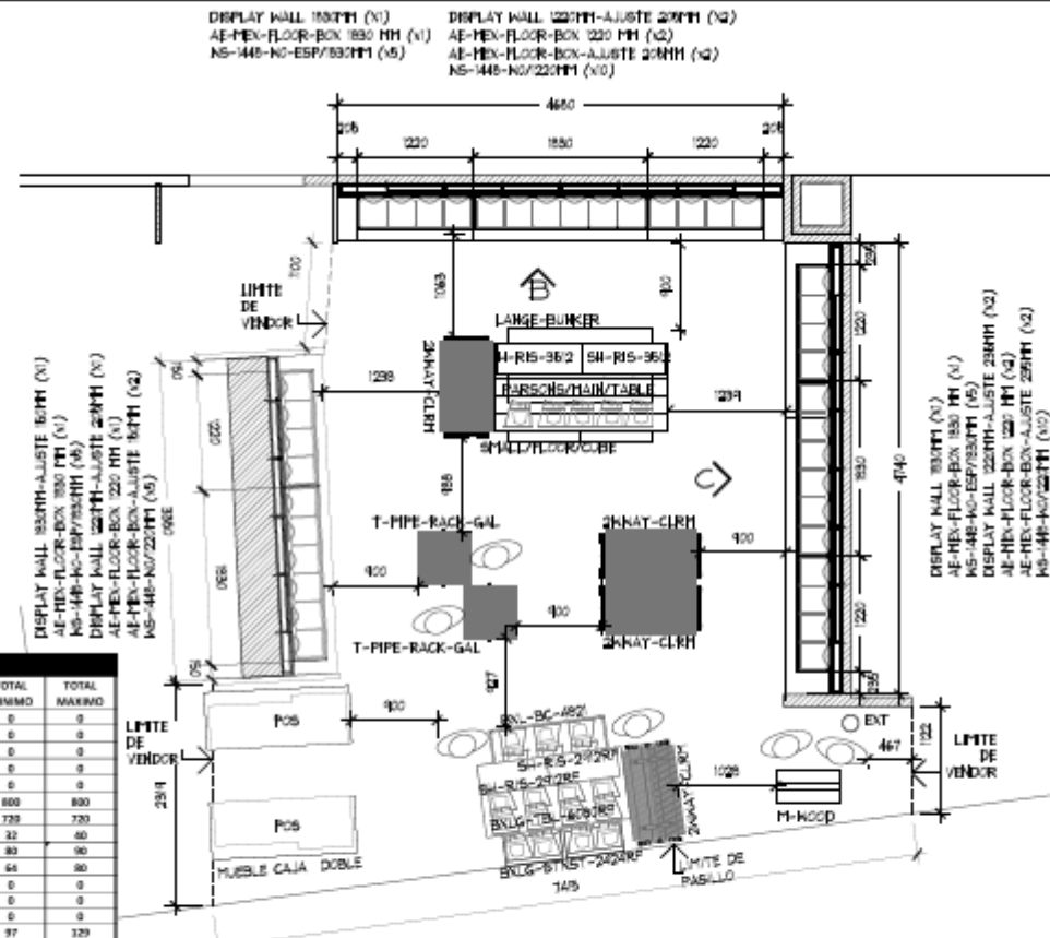
PLANTA ARQUITECTONICA
