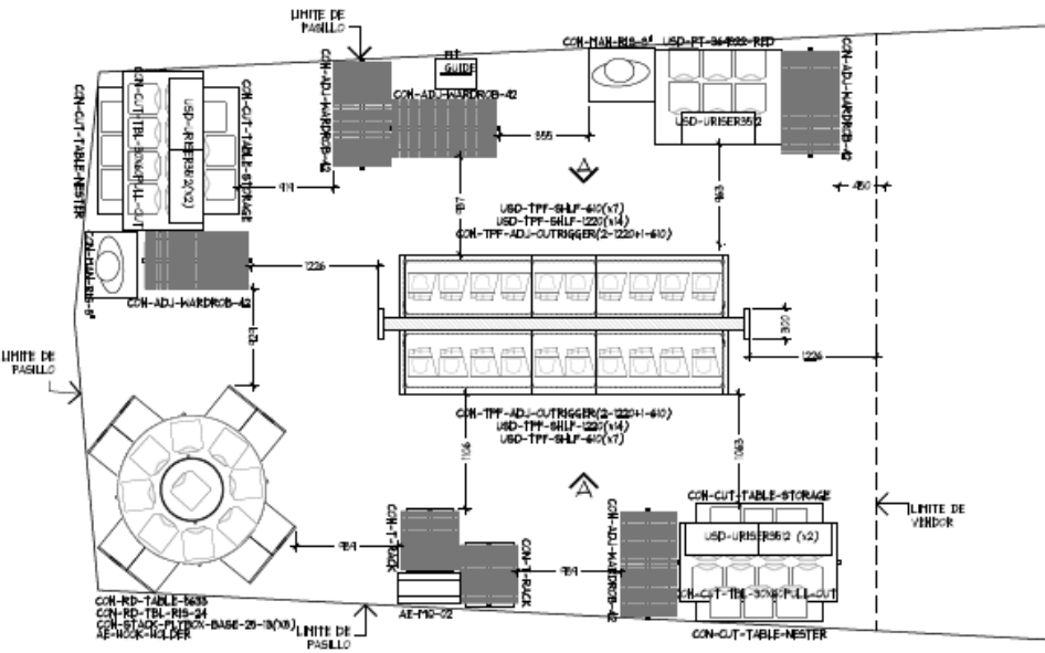
PLANTA MOBILIARIO ESC. 1:50
