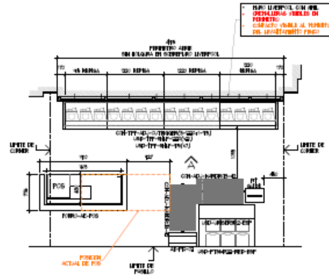
PLANTA ARQUITECTONICA ESC. 1:50
