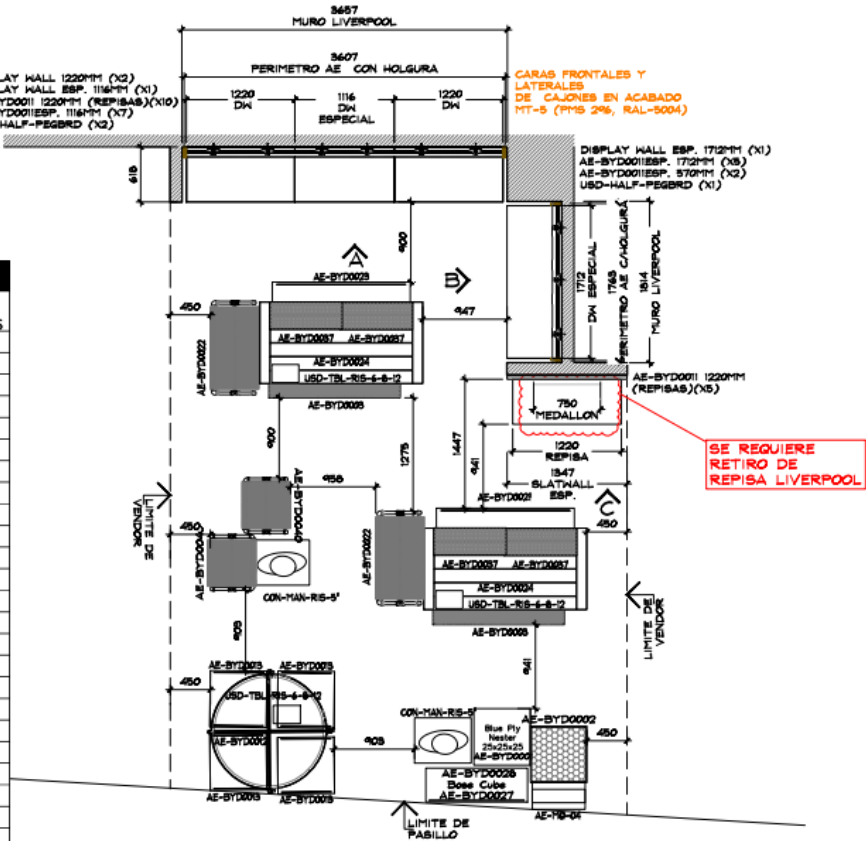
PLANTA MOBILIARIO ESC. 1:50
