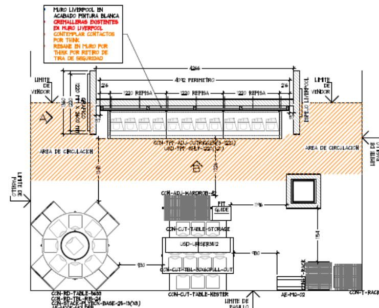
PLANTA ARQUITECTONICA ESC. 1:50
