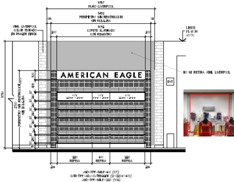
ALZADO A ESC. 1:50
