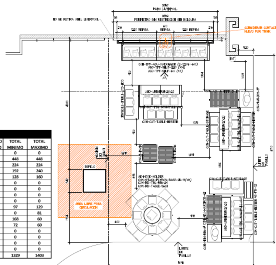
PLANTA ARQUITECTONICA ESC. 1:50
