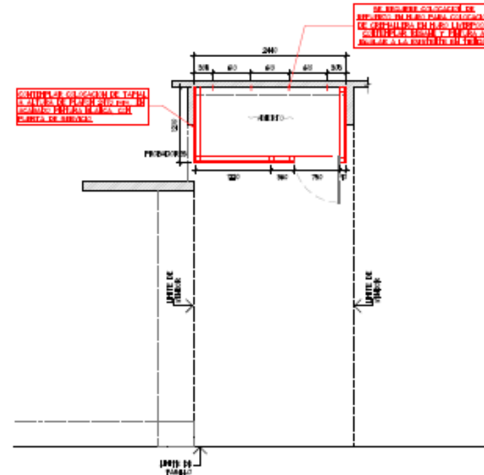
PLANTA CREMALLERAS ESC. 1:50
