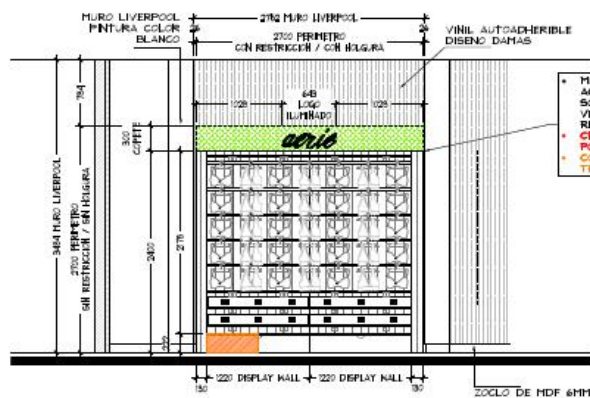
ALZADO A ESC. 1:50
