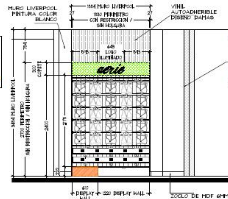
ALZADO B ESC. 1:50
