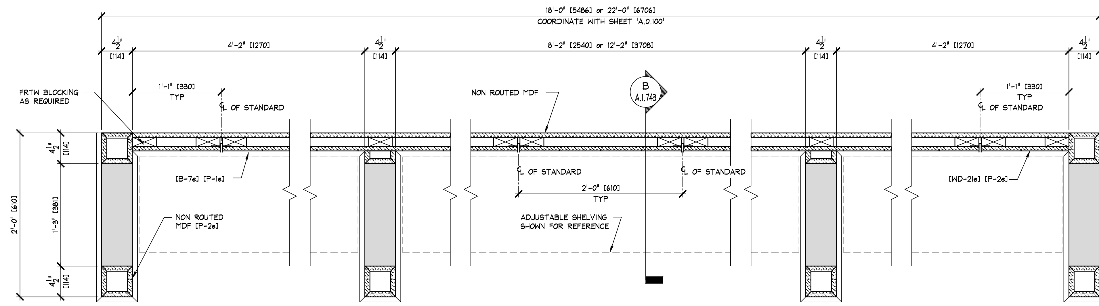
PREFAB. DISPLAY CASE ASSEMBLY 'D' PLAN SCALE: 1 1/2" = 1'-0" [1:8]
