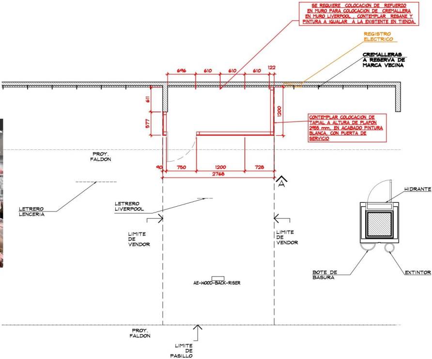
PLANTA CREMALLERAS ESC. 1:50
