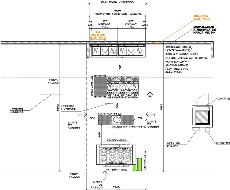
PLANTA ARQUITECTÓNICA ESC. 1:50
