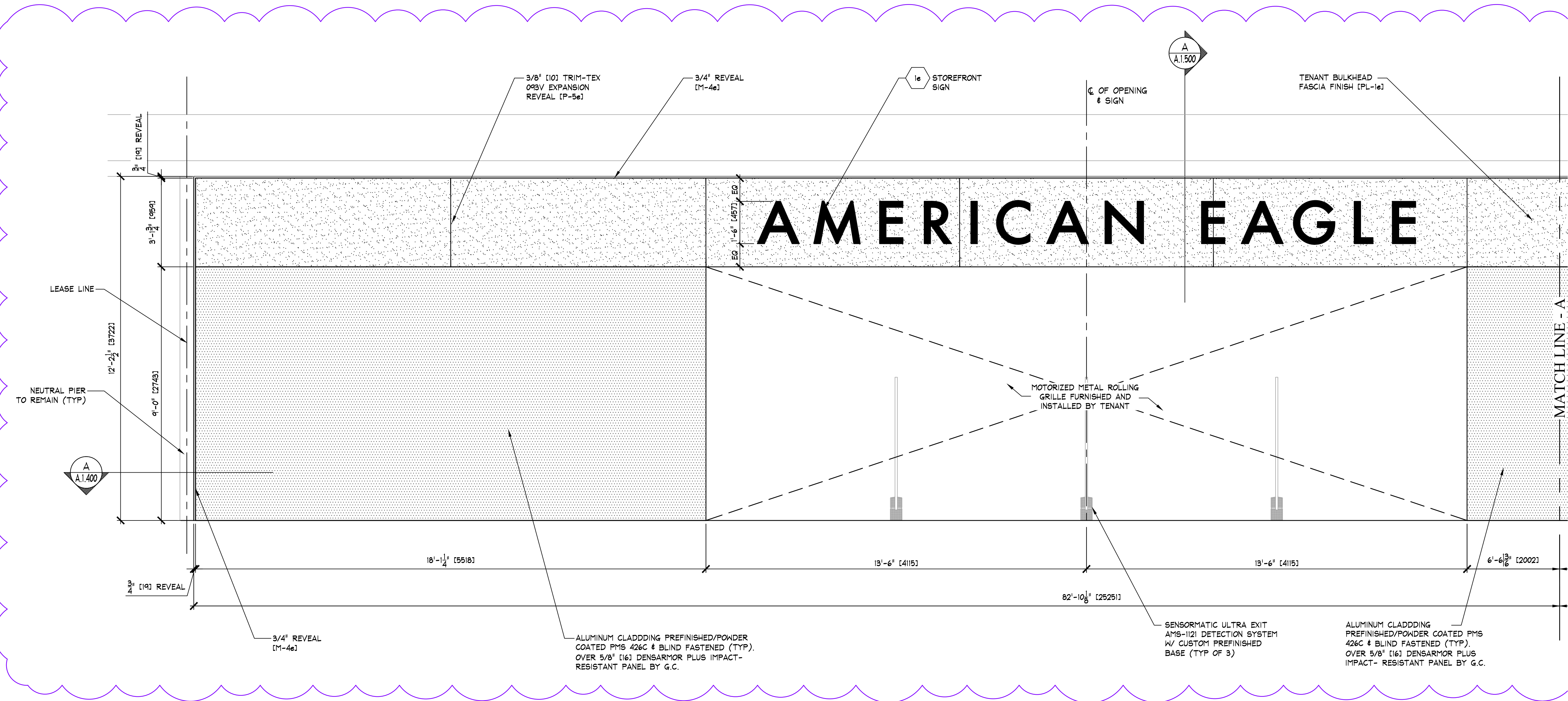
A STOREFRONT EXTERIOR ELEVATION A1.300 SCALE: 1/2" = 1'-0" (1:25)
