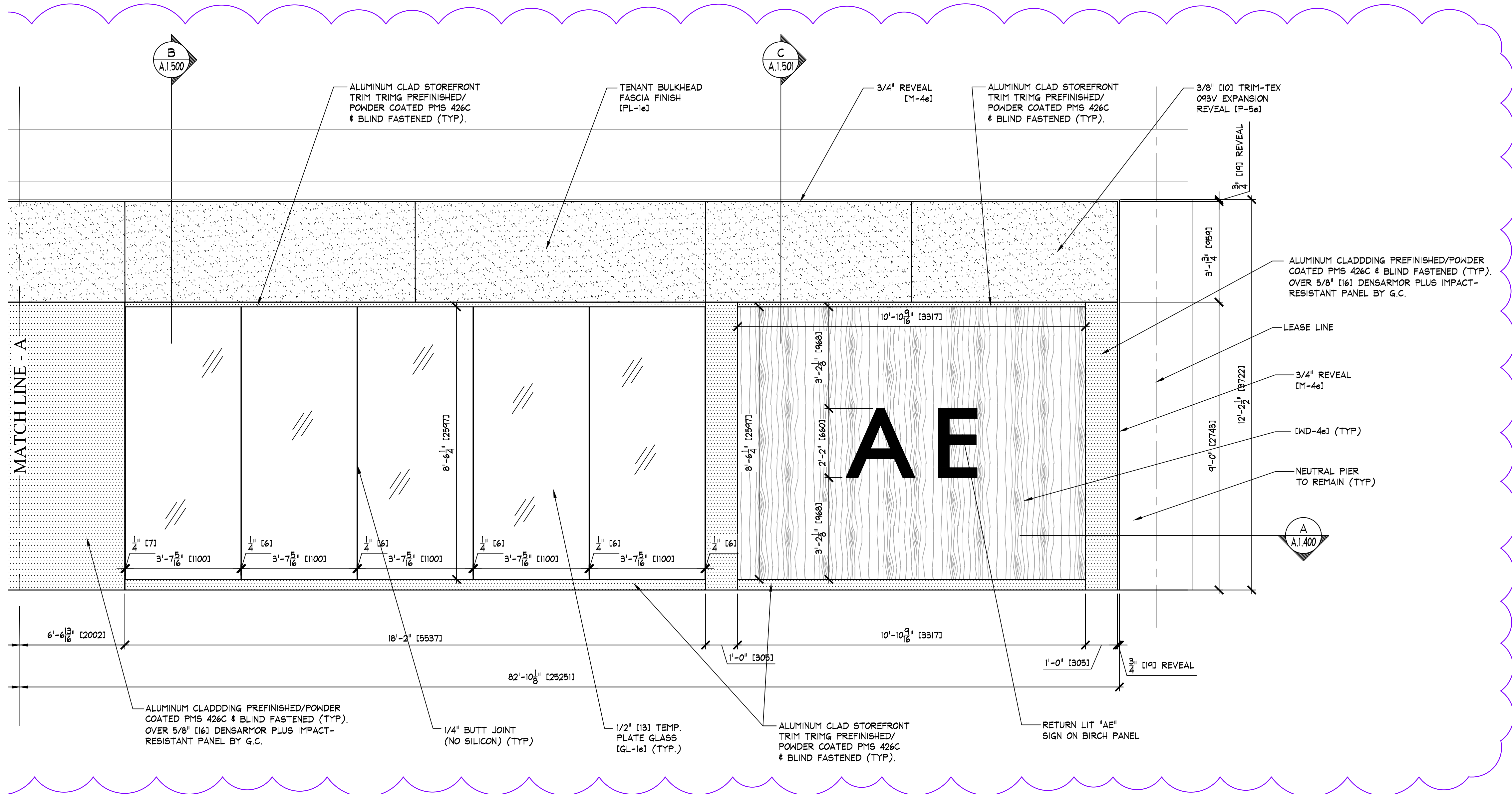
B STOREFRONT EXTERIOR ELEVATION A1.300 SCALE: 1/2" = 1'-0" (1:25)
