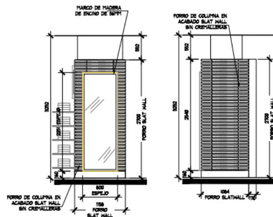
ALZADO D ESC. 1:50
