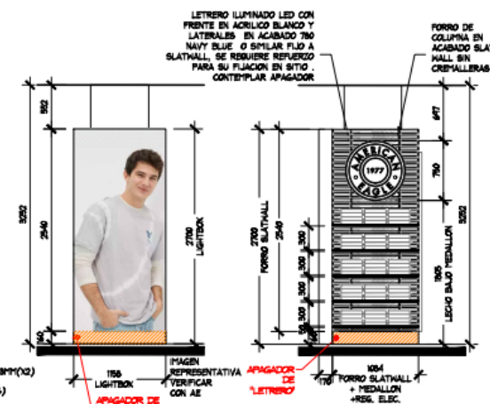
ALZADO B ESC. 1:50
