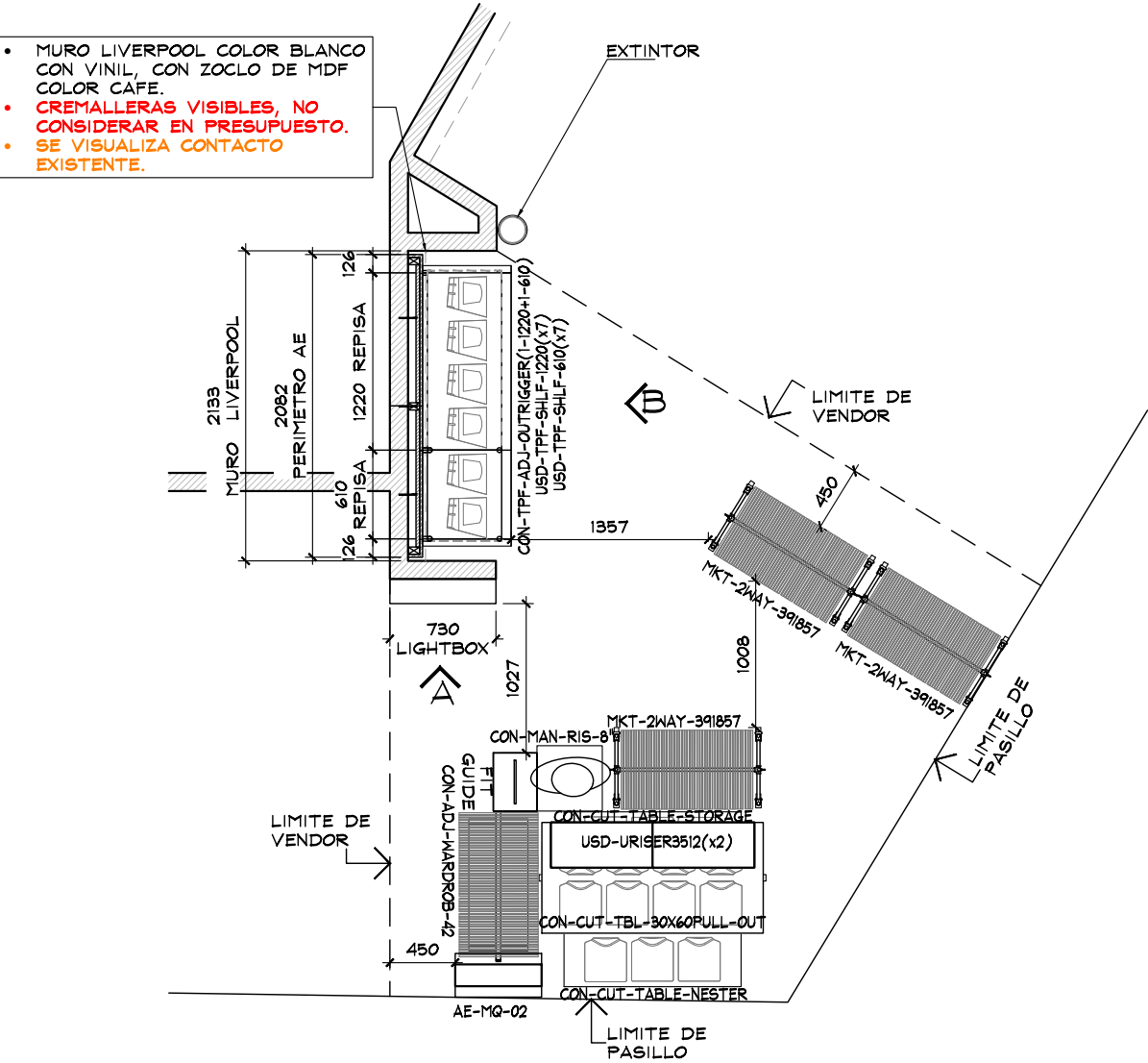
PLANTA ARQUITECTONICA ESC. 1:50
