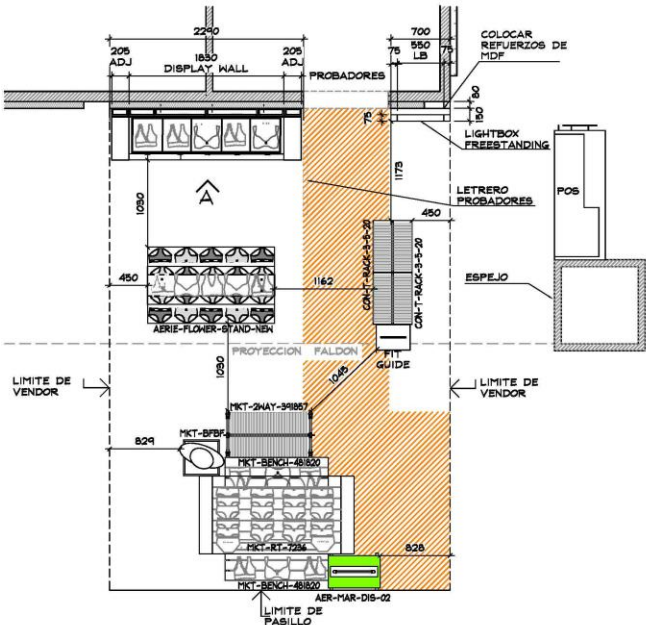
PLANTA ARQUITECTÓNICA ESC. 1:50
