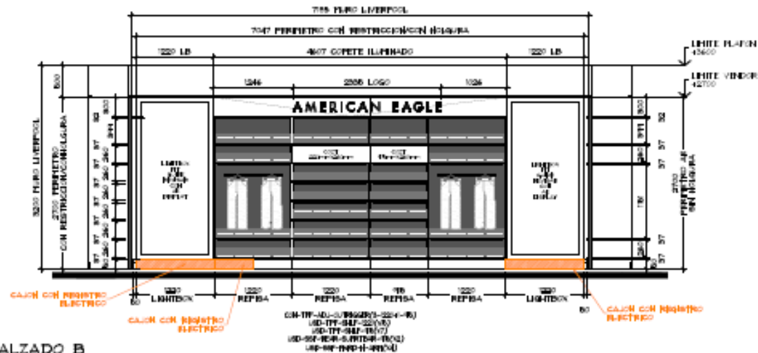
ALZADO B ESC. 1:50
