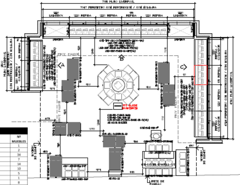
PLANTA ARQUITECTONICA EBC. 1:50
