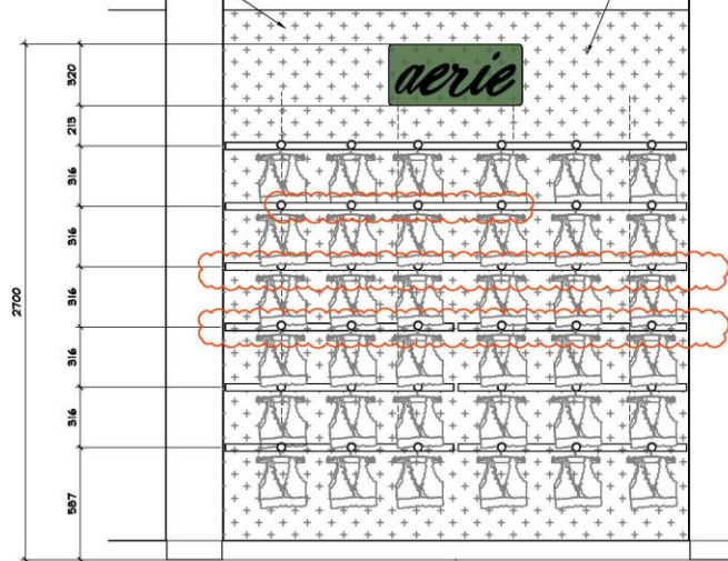
ALZADO A ESC. 1:25
