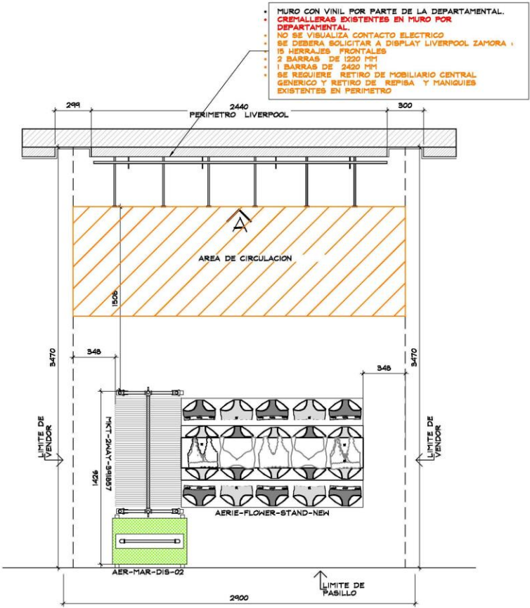
PLANTA ARQUITECTONICA ESC. 1:25
