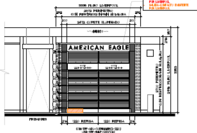
ALZADO A ESC. 1:50
