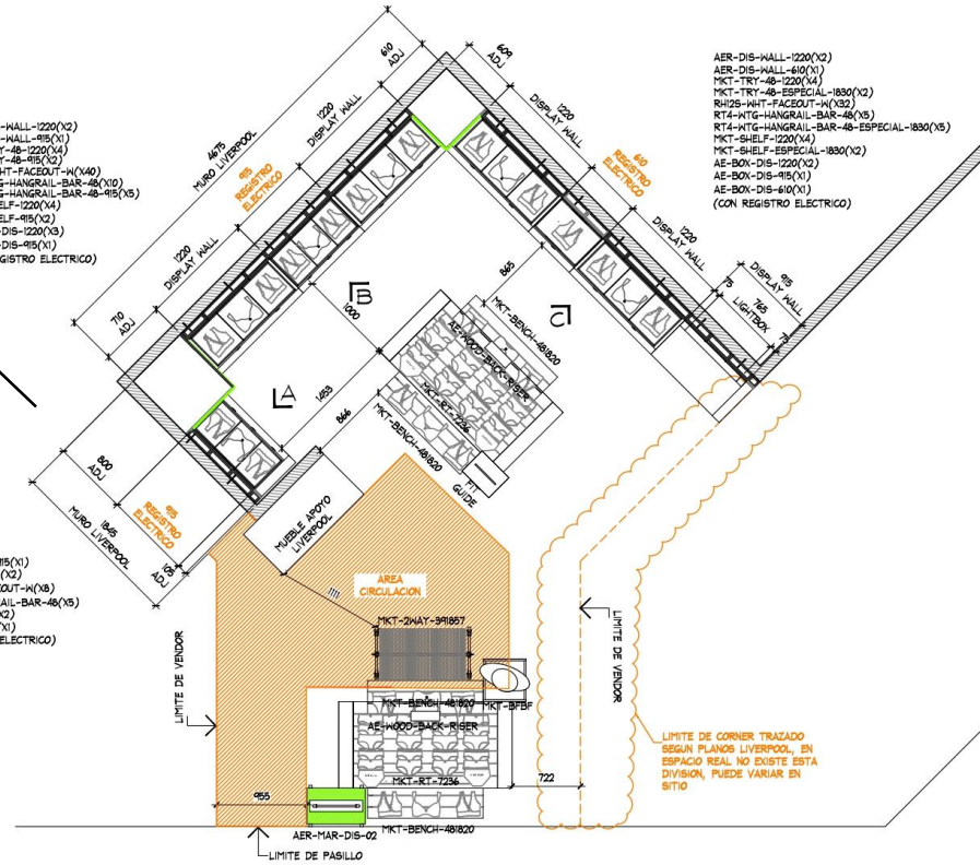
PLANTA ARQUITECTONICA ESC. 1:80
