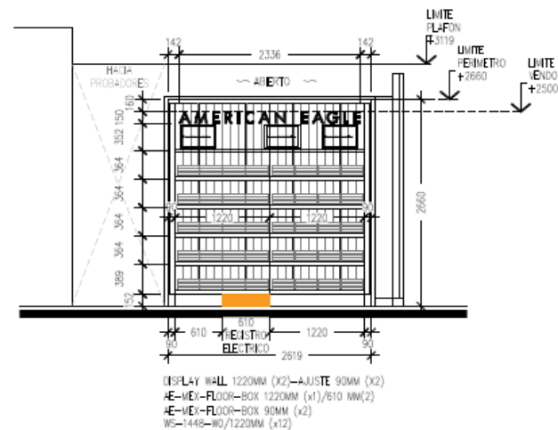
ALZADO A ESC. 1:50
