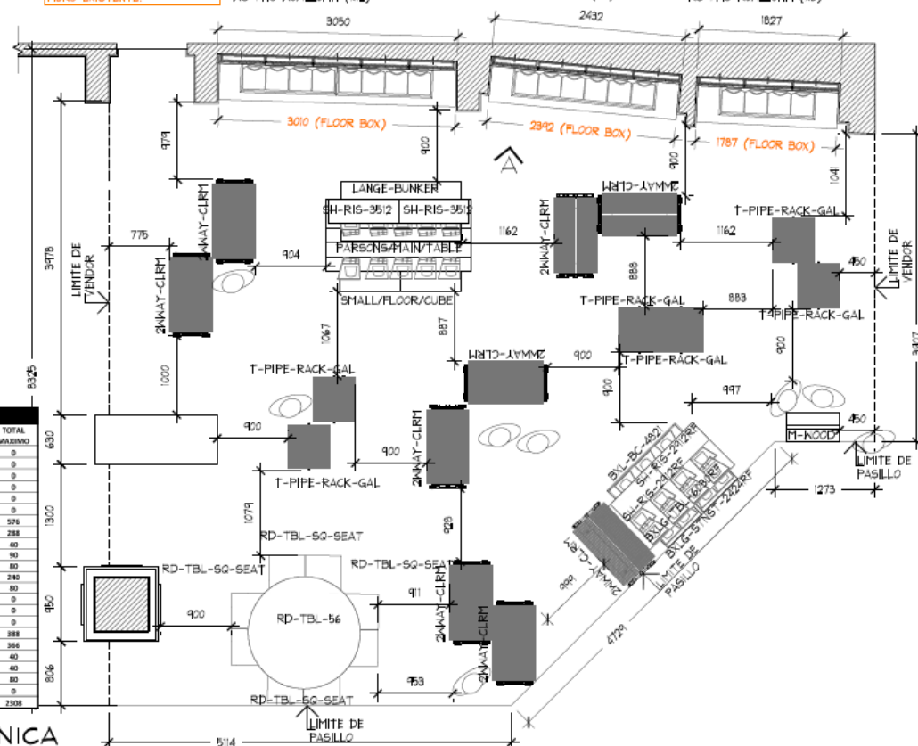
PLANTA ARQUITECTONICA
