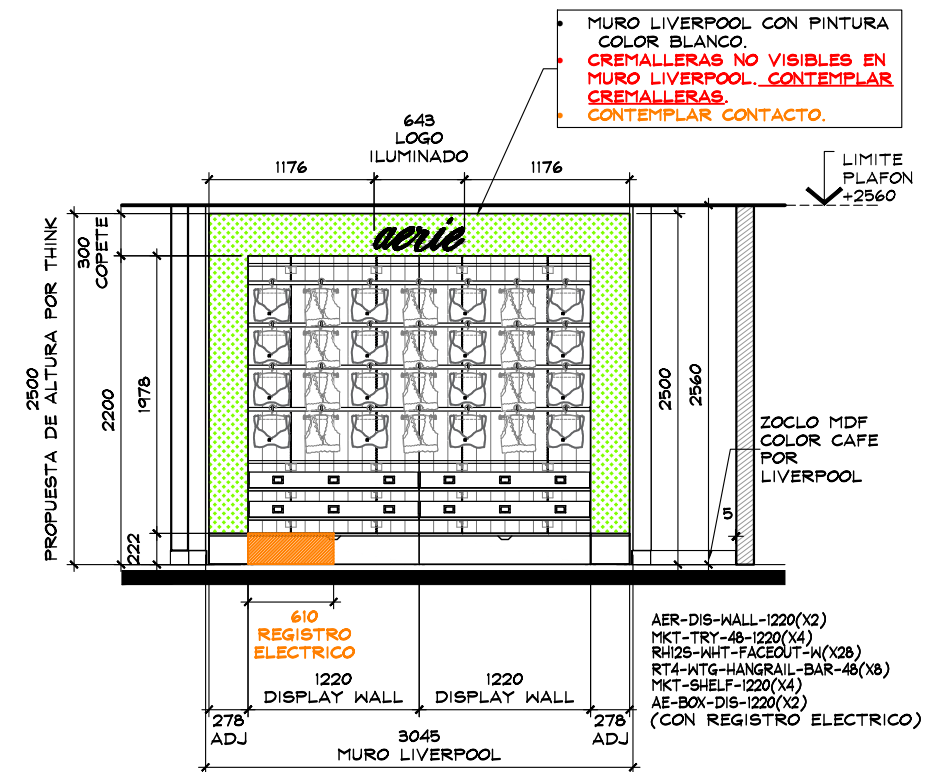
ALZADO A ESC. 1:50
