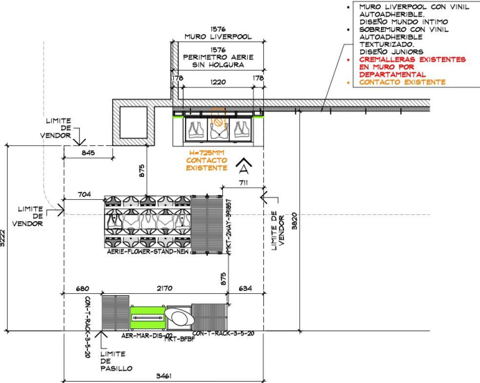
PLANTA ARQUITECTONICA ESC. 1:50
