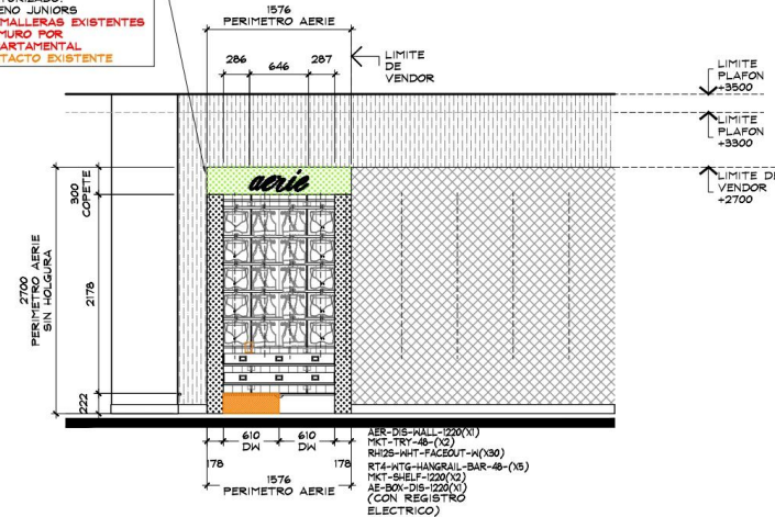
ALZADO A ESC. 1:50
