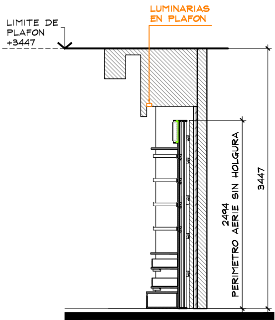
CORTE A ESC. 1:50
