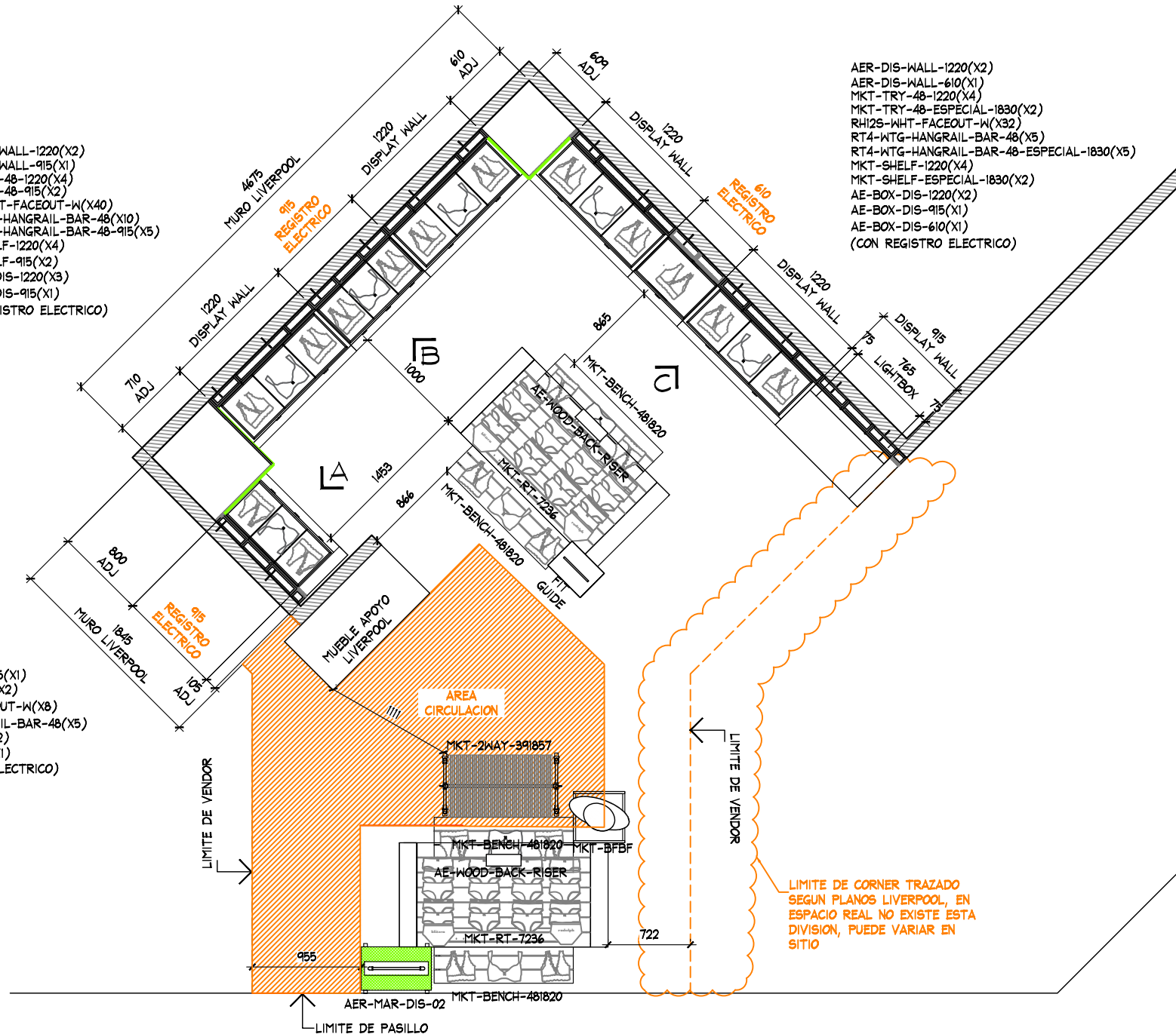
PLANTA ARQUITECTONICA EBC. 1:50
