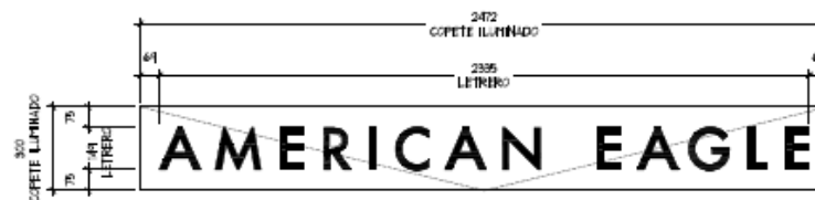
DETALLE LOGO ESC. 1:20
