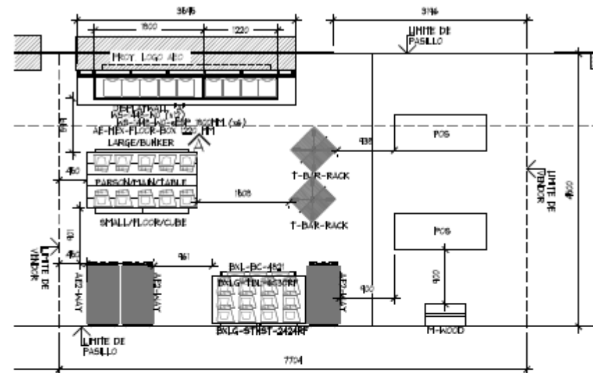
PLANTA ARQUITECTONICA
