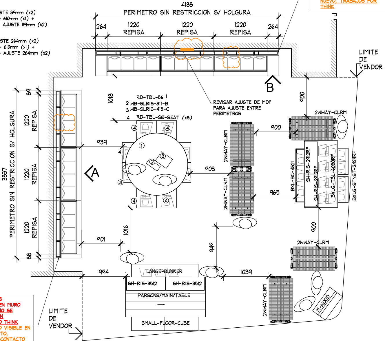
PLANTA ESC. 1:50
