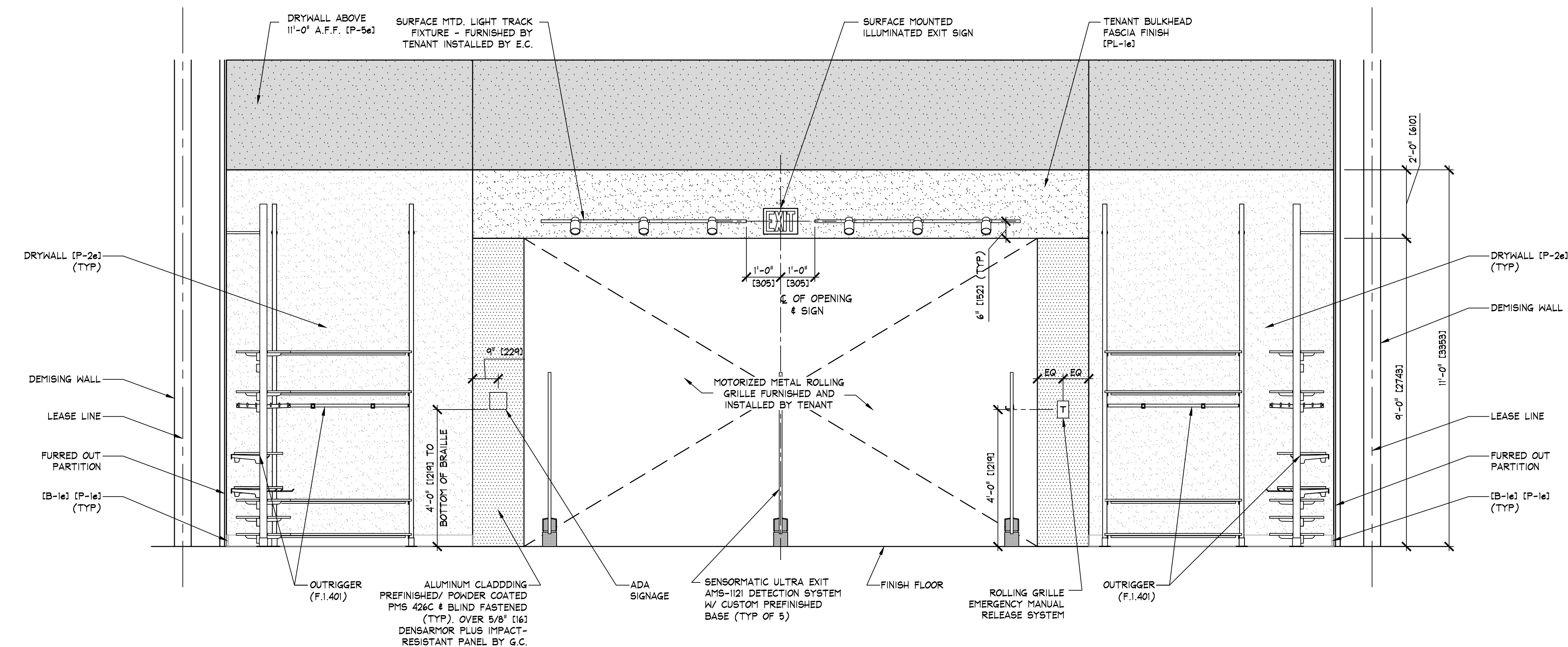
B STOREFRONT INTERIOR ELEVATION A.1.300 SCALE: 1/2" = 1'-0" (1.25)
