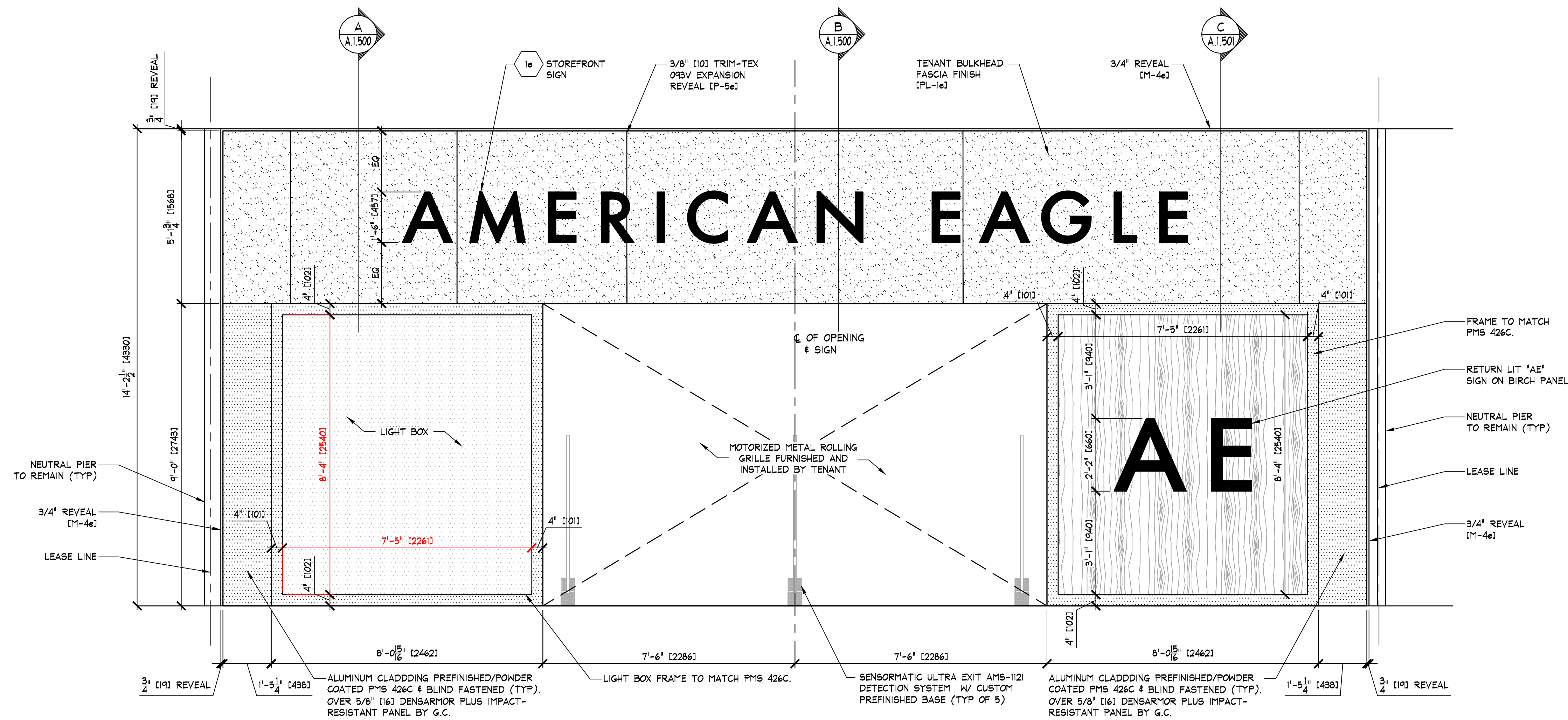
A STOREFRONT EXTERIOR ELEVATION A.1.300 SCALE: 1/2" = 1'-0" (1.25)
