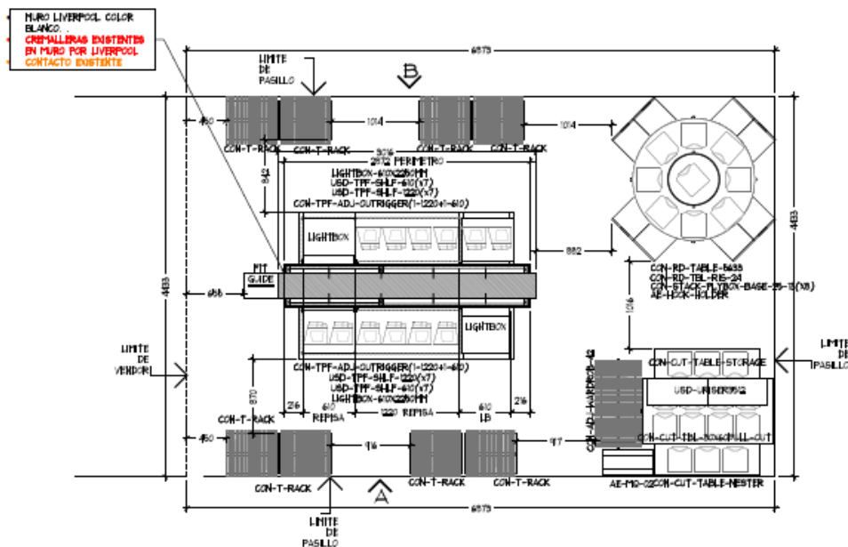
PLANTA ARQUITECTONICA ESC. 1:50
