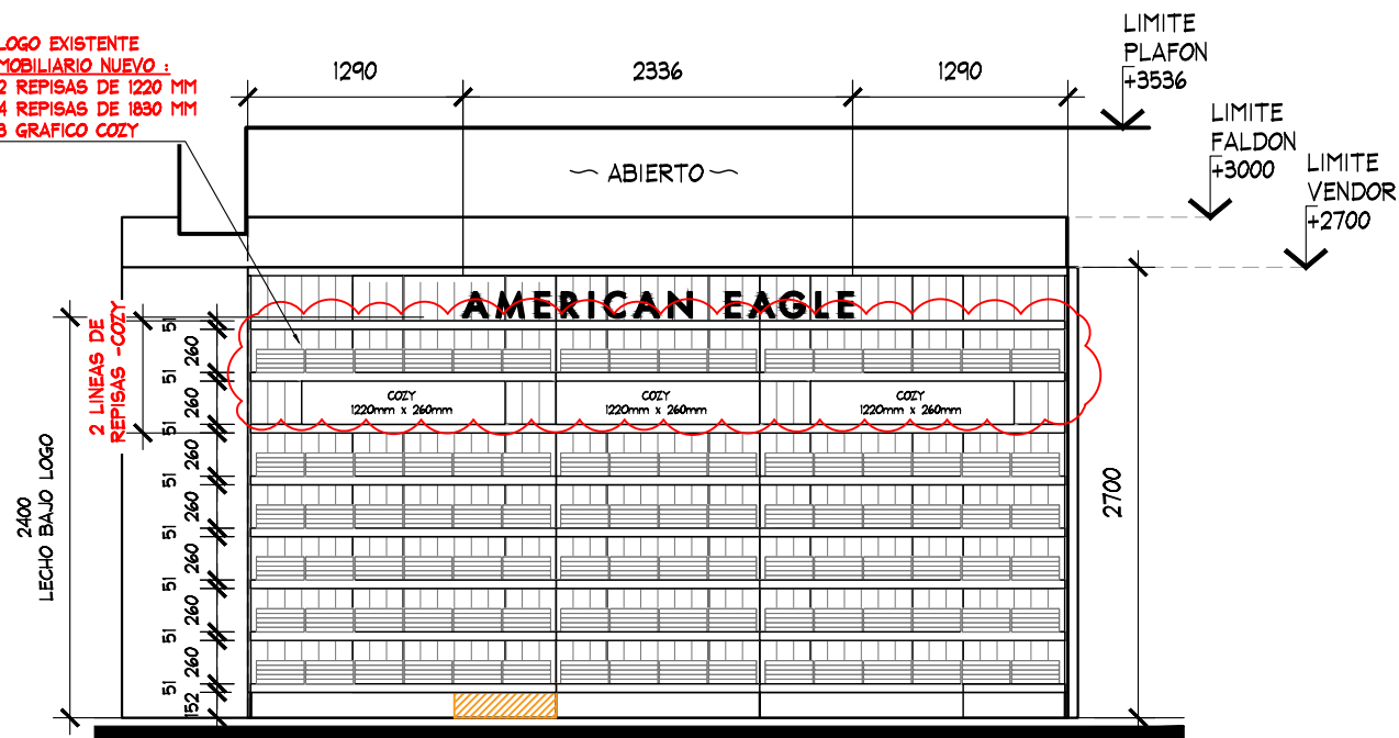
ALZADO A ESC. 1:50
