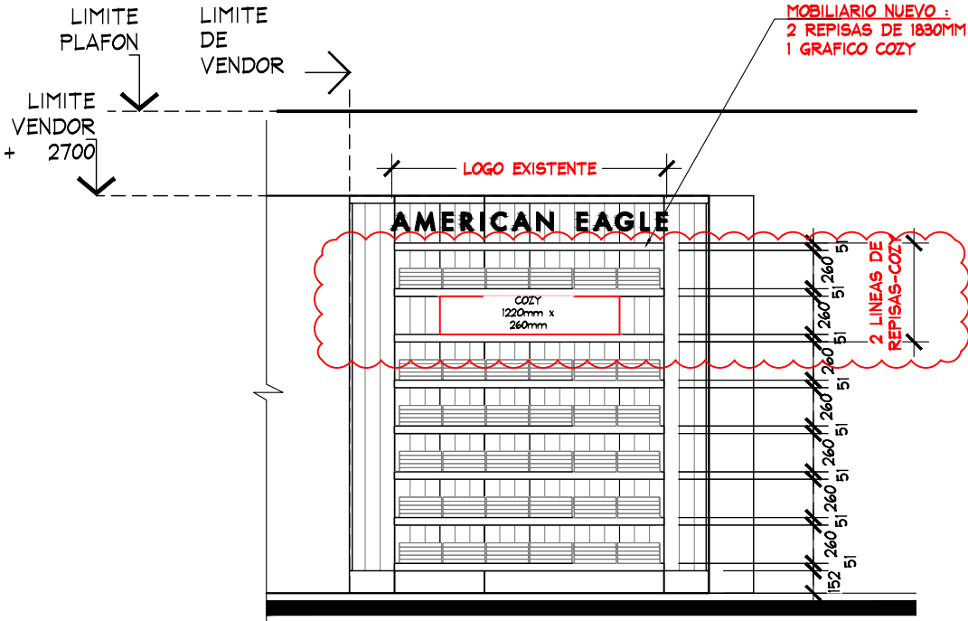
ALZADO "A" ESC. 1:50
