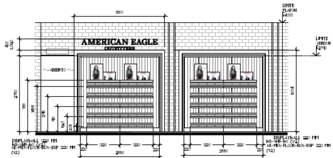
ALZADO A ESC. 1:50
