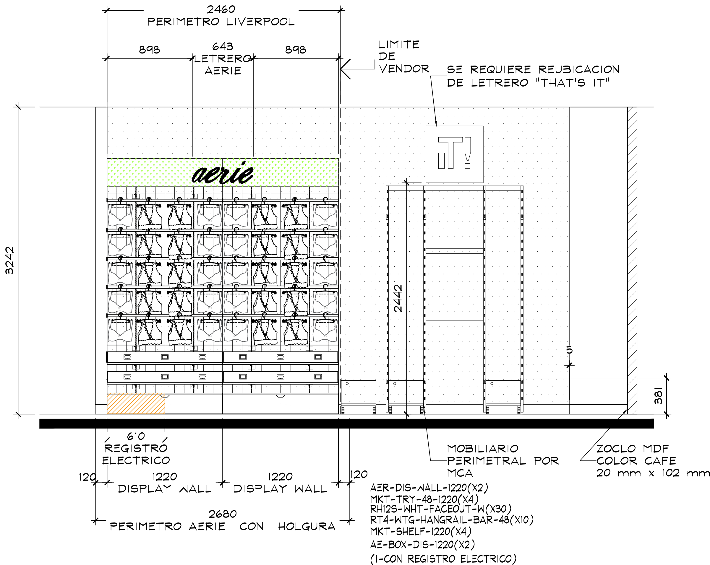
ALZADO A ESC. 1:50
