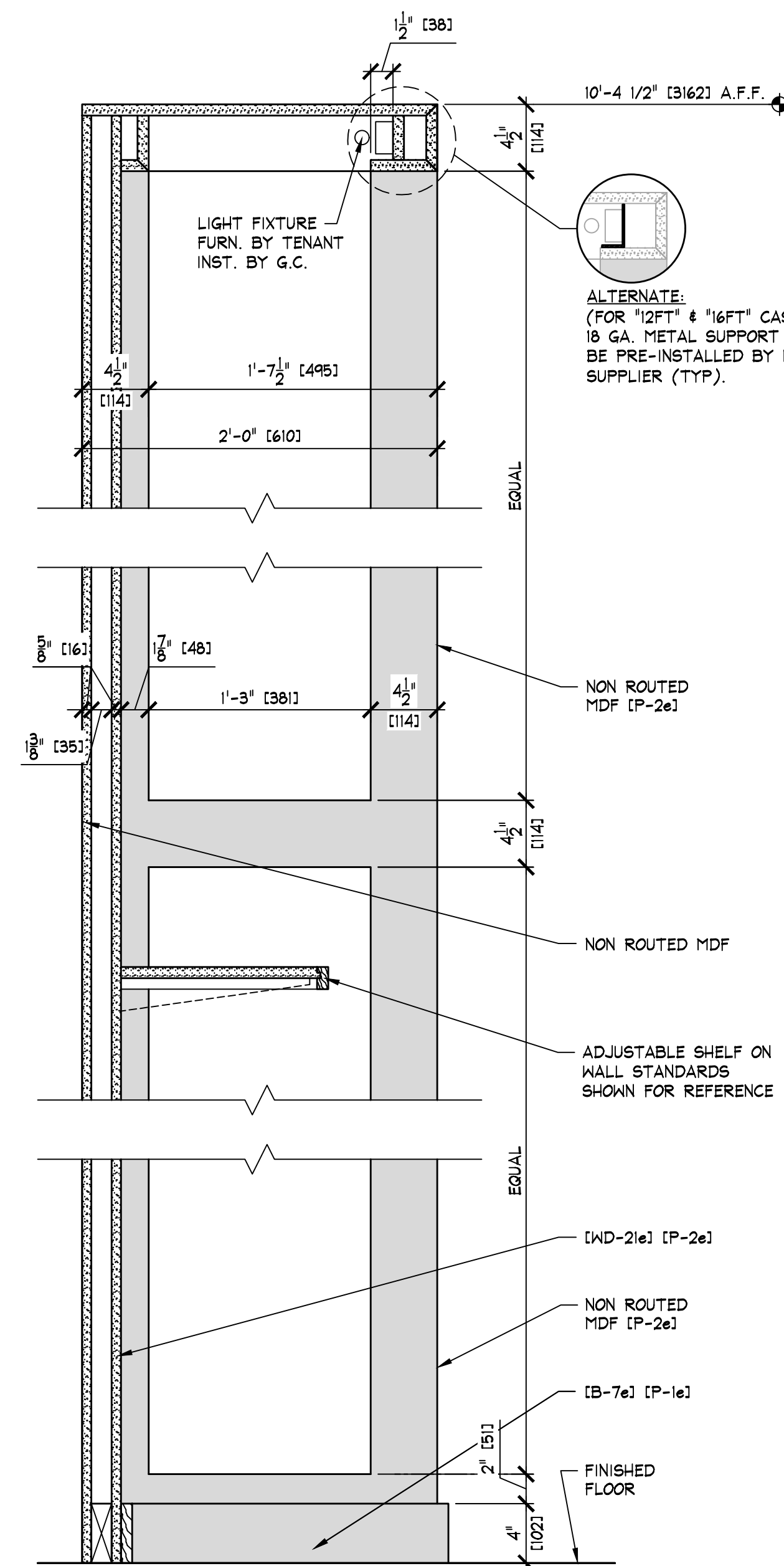
PREFAB. DISPLAY CASE ASSEMBLY 'B' SECTION SCALE: 1 1/2" = 1'-0" (1:8)
