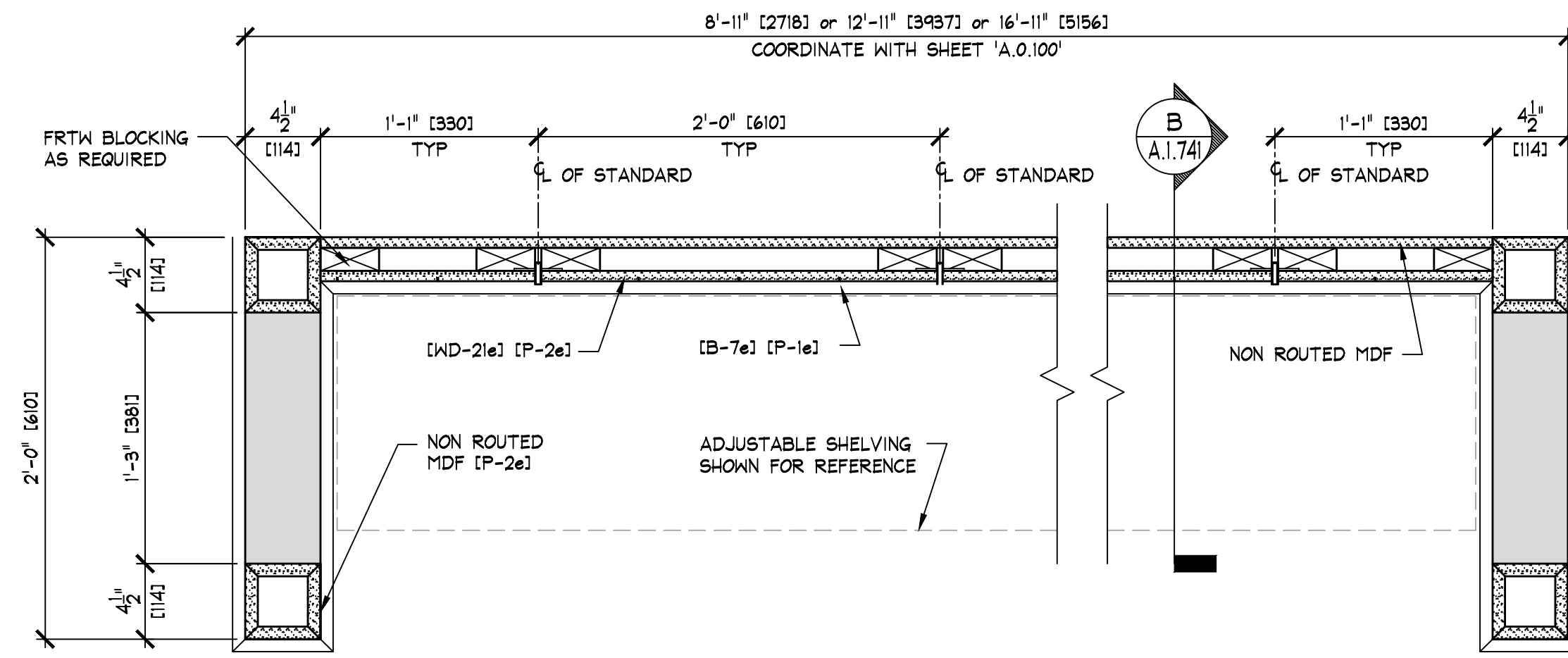
PREFAB. DISPLAY CASE ASSEMBLY 'B' PLAN SCALE: 1 1/2" = 1'-0" (1:8)
