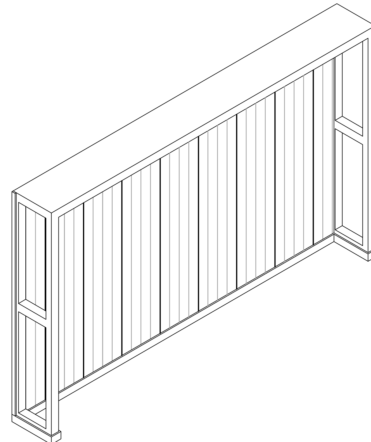
PREFAB. DISPLAY CASE ASSEMBLY 'B' PERSPECTIVE SCALE: N.T.S.
