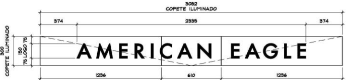
DETALLE DE LETRERO ESC. 1:20
