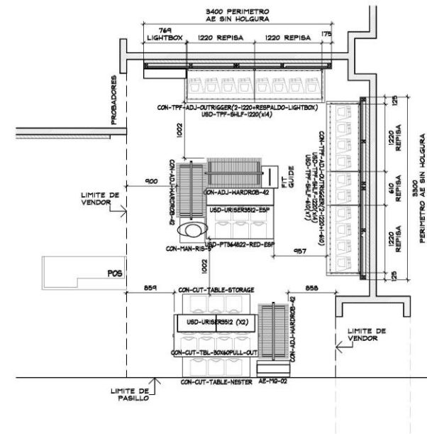
PLANTA ARQUITECTONICA ESC. 1:50
