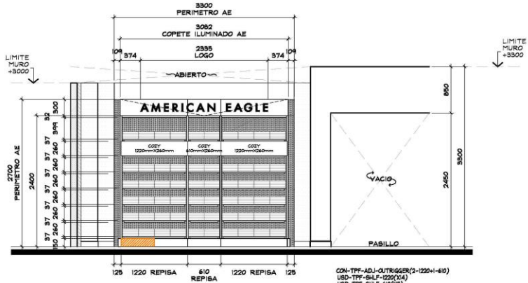
ALZADO B ESC. 1:50
