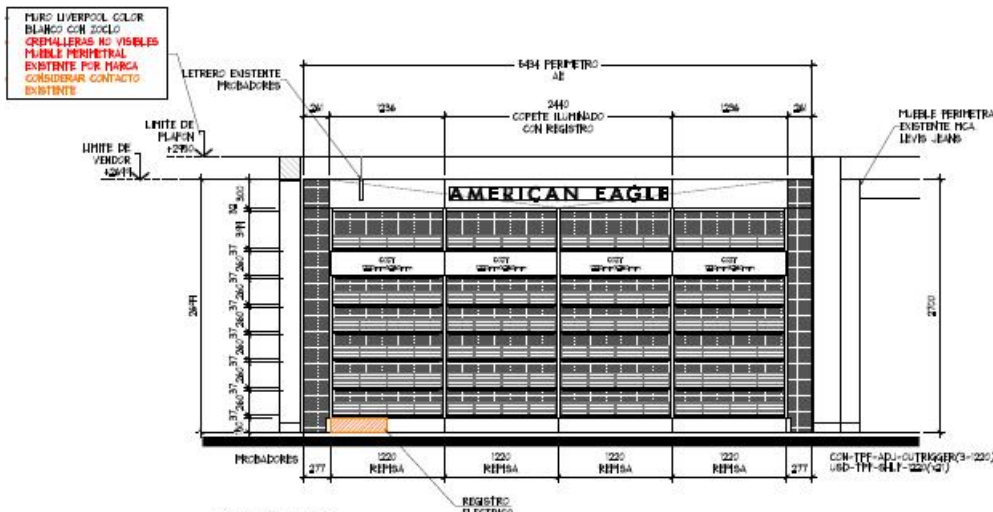
ALZADO B ESC. 1:50
