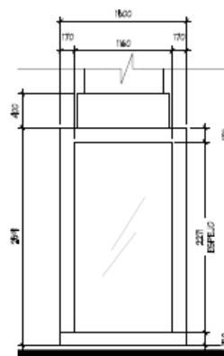
ALZADO C
