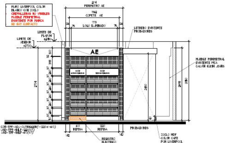
ALZADO A ESC. 1:50
