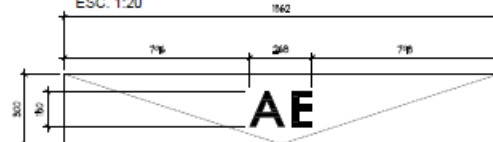
DETALLE LETRERO
