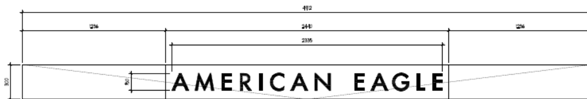
DETALLE LETRERO
