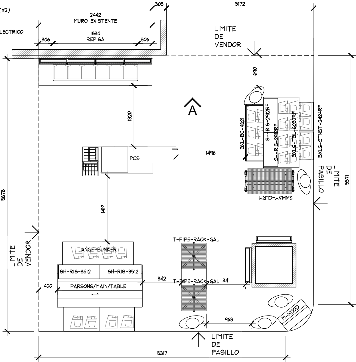
PLANTA DE MOBILIARIO ESC. 1:50
