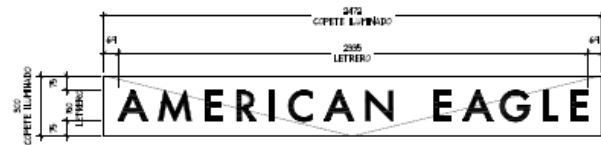
DETALLE LOGO 1/2 ESC. 1:20
