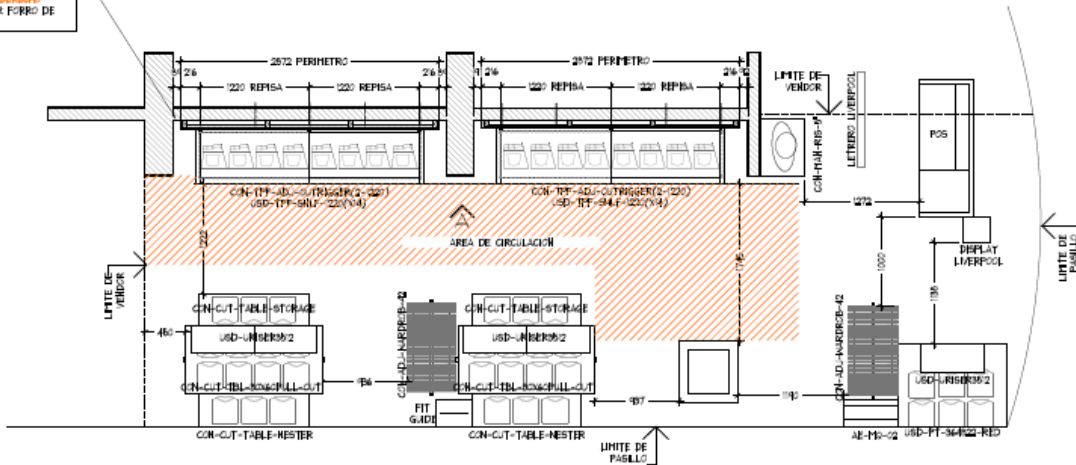
PLANTA ARQUITECTONICA ESC. 1:50
