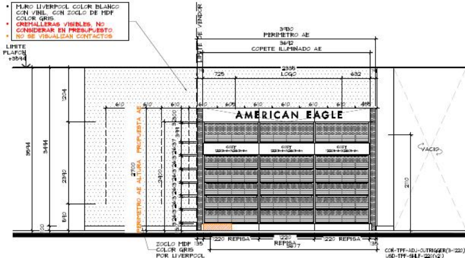
ALZADO A ESC. 1:50
