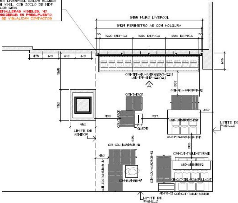
PLANTA DE ARQUITECTONICA ESC. 1:50
