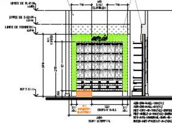
ALZADO A ESC. 1:50
