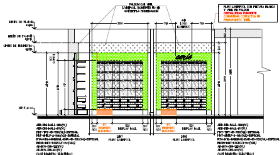
ALZADO B ESC. 1:50
