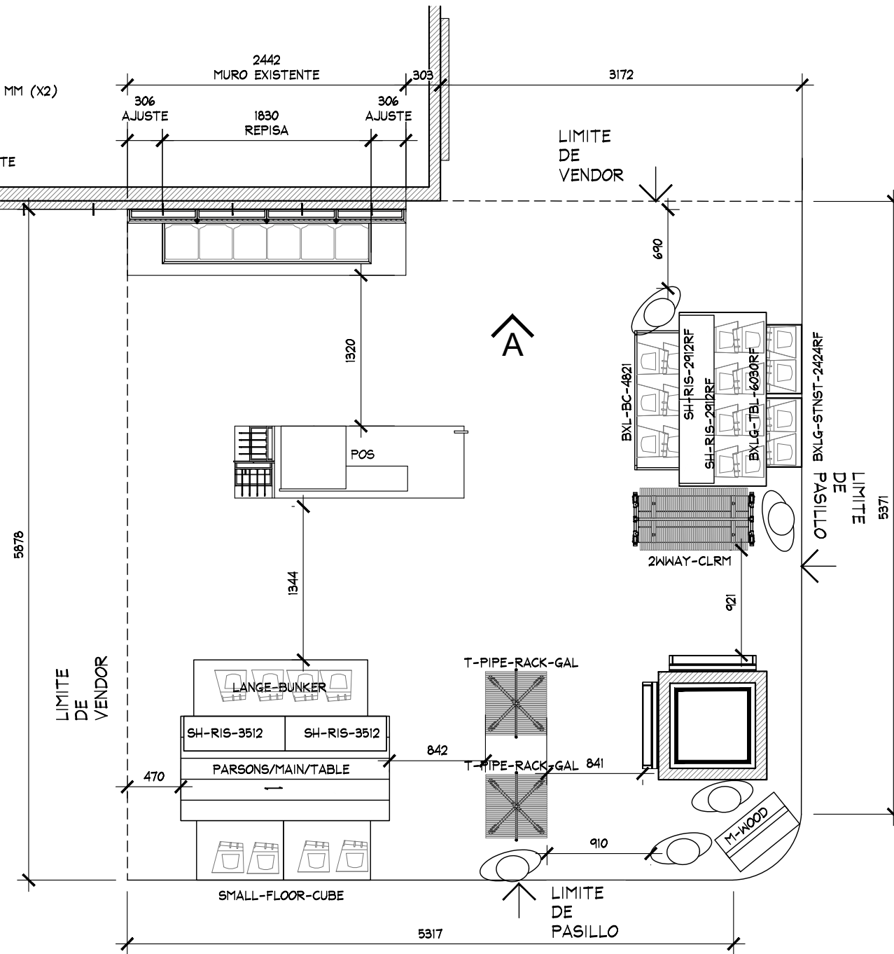
PLANTA DE MOBILIARIO ESC. 1:50
